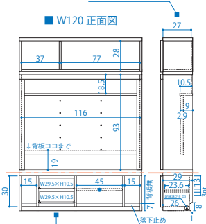
■ W120 正面図 D32タイプ側面図 (W100/120/140 共通)
