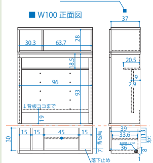
■ W100 正面図 D42タイプ側面図 (W100/120/140 共通)
