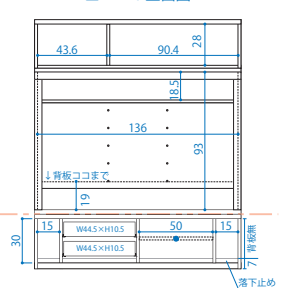
■ W140 正面図
