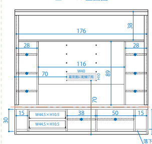
■ W180 正面図
