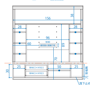
■ W160 正面図
